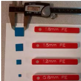
Muestras de cinta transportadora MD junto a las muestras de prueba equivalentes.
