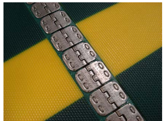
Detalle de la Aster 22AF-ski empalmada con grapa.
